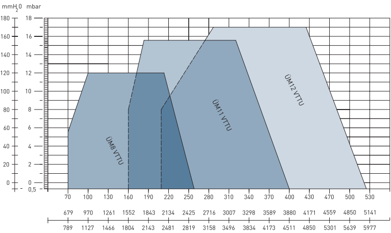
Courbes de capacité de brûleur contre la contre-pressure de chambre de combustion
