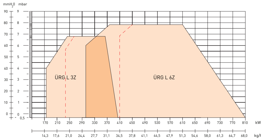
Üret İki Kademeli Çift Yakıtlı Brülörler Kapasite Tablosu / Capacity Table of Üret Two Stage Dual Burners
